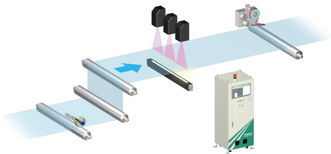
Mujiken Express システム構成
